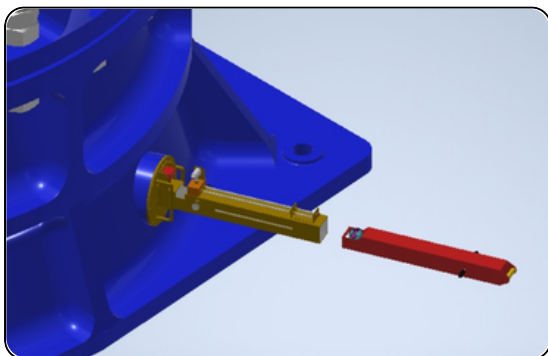
Instalación del Bottom Scan en la chancadora
